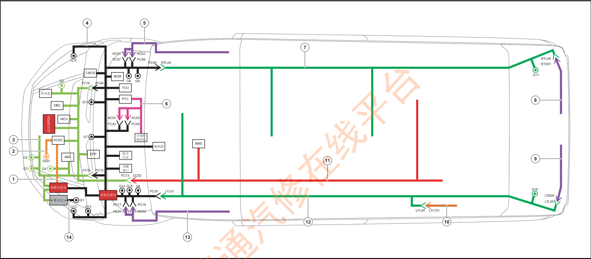
低压电路布置说明
